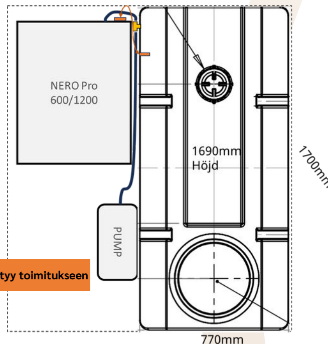
Esimerkkiasennus 1600 L säiliölle
