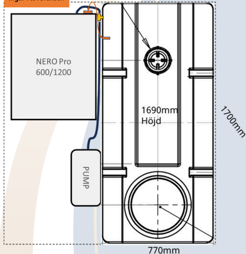
Exempel installation med PRO 1600 L tank
